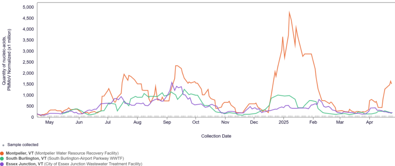
SARS-CoV-2, Vermont
